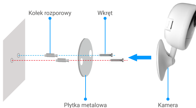
Rys.2 Mocowanie za pomocą wkrętów
